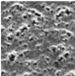
Surface lisse d'un profil PVC extrudé de manière habituelle (image au microscope).
